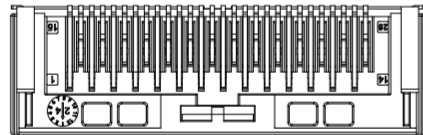
28PIN 2069W-F2804-XXF09
