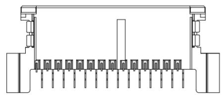
28PIN 2069W-F2804-XXF06
